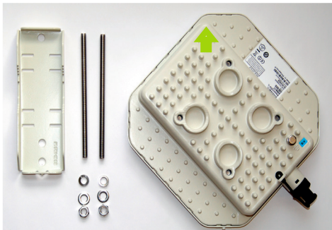
Montagematerial & Antennenrückseite
