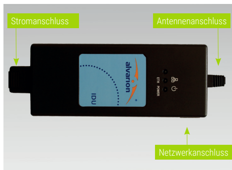
Netzteil (IDU) mit Strom-, Antenne- und Netzwerkanschluss
