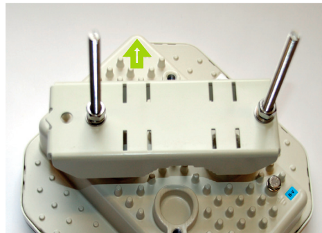
Montierte Haltevorrichtung
